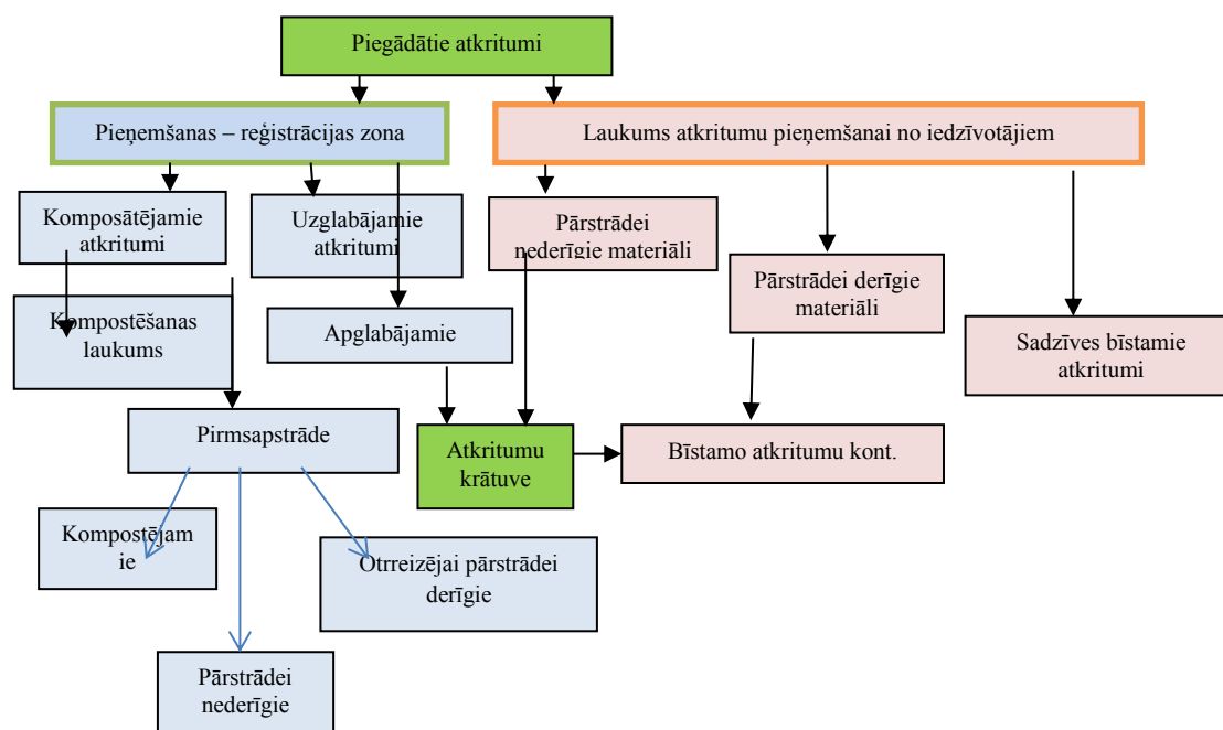
Attēls Nr.2 Poligonā „Ciniši” piegādāto atkritumu plūsmas shēma
